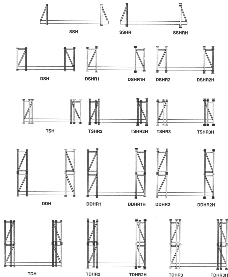
MU-Brücke – Aufbautypen, je nach Spannweite und Belastung
